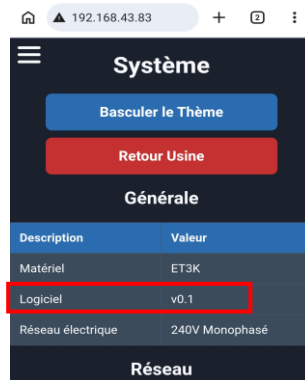
Figure 11 : Version logicielle
